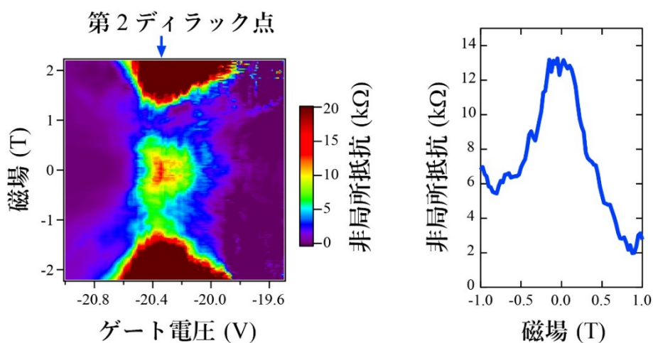
図4: バレー流生成に対応する巨大な非局所抵抗シグナル
