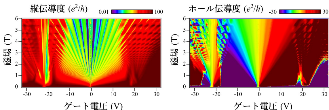
図3: 量子ホール効果と超格子構造に対応する'蝶'
