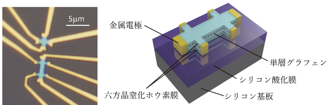
図2: グラフェンと六方晶窒化ホウ素で作製した原子層超格子デバイス
